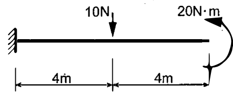
図1(b) 梁B
