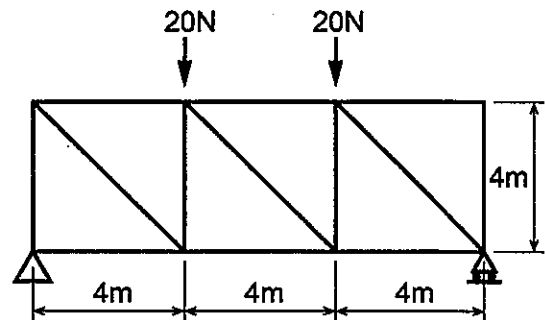
図2 トラス架構
