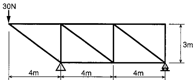
図2 トラス架構
