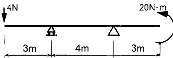
図1(a) 梁A
