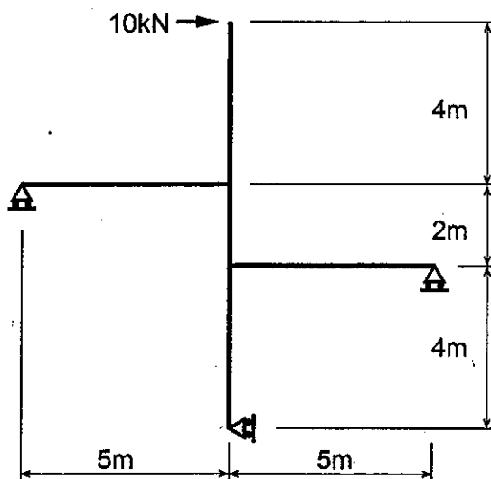
図3 架構A
